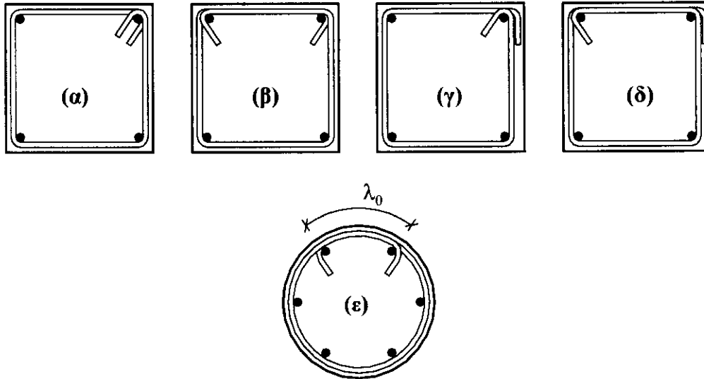
Σχήμα 17.5: Κλείσιμο συνδετήρων σε κορμούς πλακοδοκών, σε δοκούς, σε υποστρώματα και τοιχώματα (βλ. Σχήμα 17.3 για αγκύρωση άκρων)
